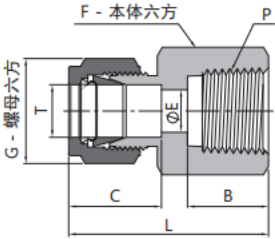
卡套阴螺纹接头
