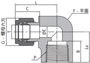
卡套阴螺纹弯头
