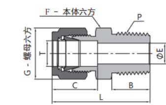
卡套阳螺纹接头
