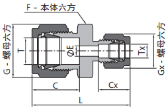
卡套直通变径接头
