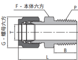
卡套阳螺纹镗通接头
