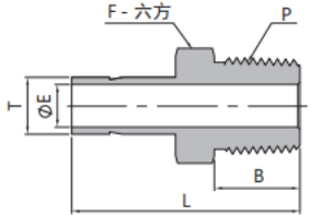
卡套管-阳螺纹
