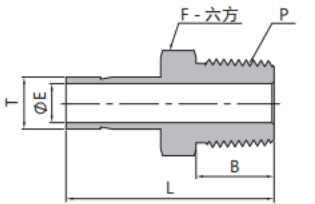
卡套管-阳螺纹
