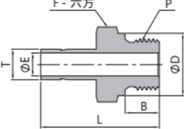
卡套管-阳螺纹
