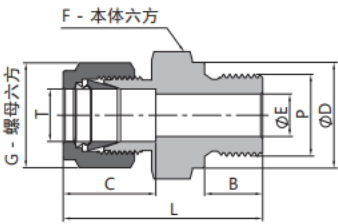
卡套阳螺纹接头
