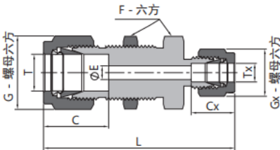
卡套直通穿板变径接头
