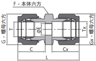
卡套直通转换接头
