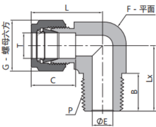
卡套阳螺纹弯头
