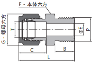
卡套阳螺纹接头
