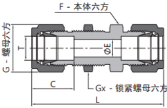
卡套直通穿板接头
