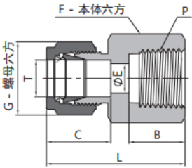
卡套阴螺纹接头
