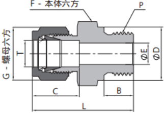
卡套阳螺纹接头
