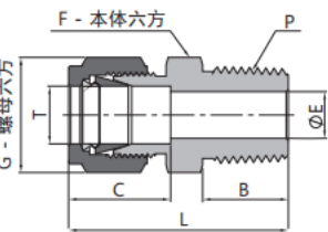
卡套阳螺纹接头
