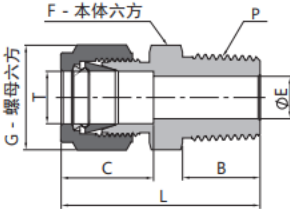
卡套阳螺纹接头
