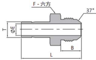
卡套管-阳螺纹
