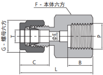
卡套阴螺纹接头
