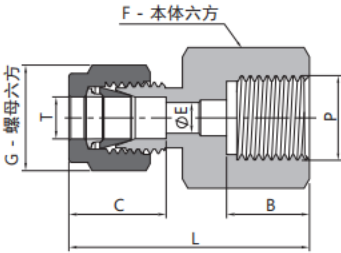
卡套阴螺纹接头
