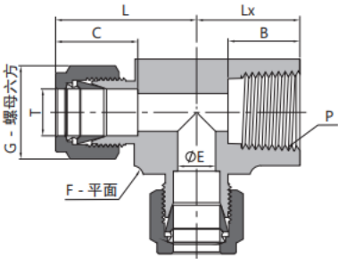
主管阴螺纹卡套三通
