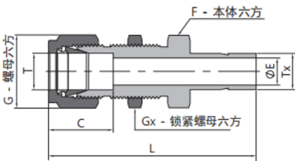
卡套穿板-卡套管
