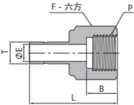
卡套管-阴螺纹
