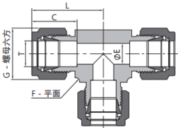
卡套三通
