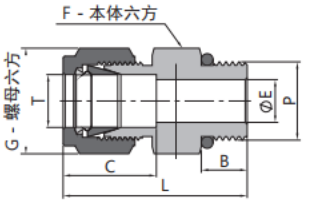
卡套阳螺纹接头
