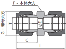
卡套直通接头
