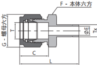
卡套-卡套管
