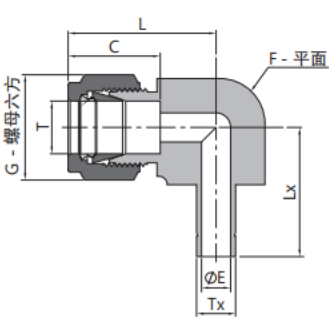
卡套-卡套管弯头
