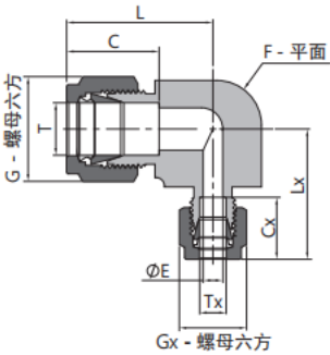
卡套变径弯头
