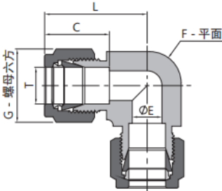
卡套弯头
