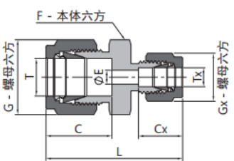
卡套直通变径接头
